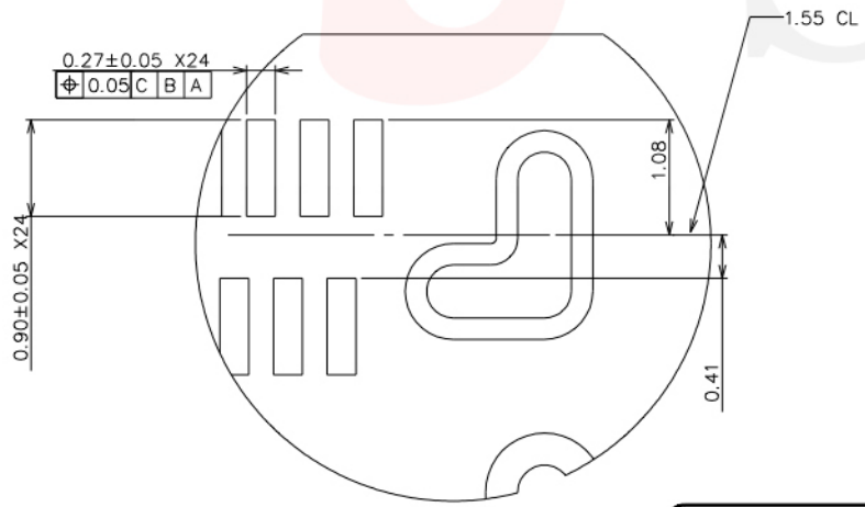
細部放大圖 A 比例 20 : 1
