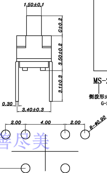
安装图 (PCB LAYOUT PLAN)
