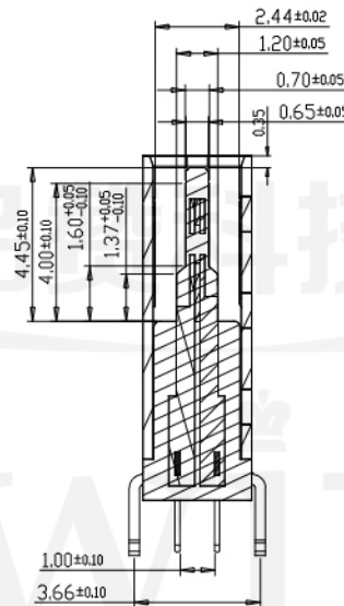
截面 1-1
